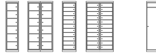
Tøyutleveringsskap med 6/11 rom i høyden. 44x50x190cm (bxdxh) Skittentøyskap 44x50x190cm (bxdxh)
